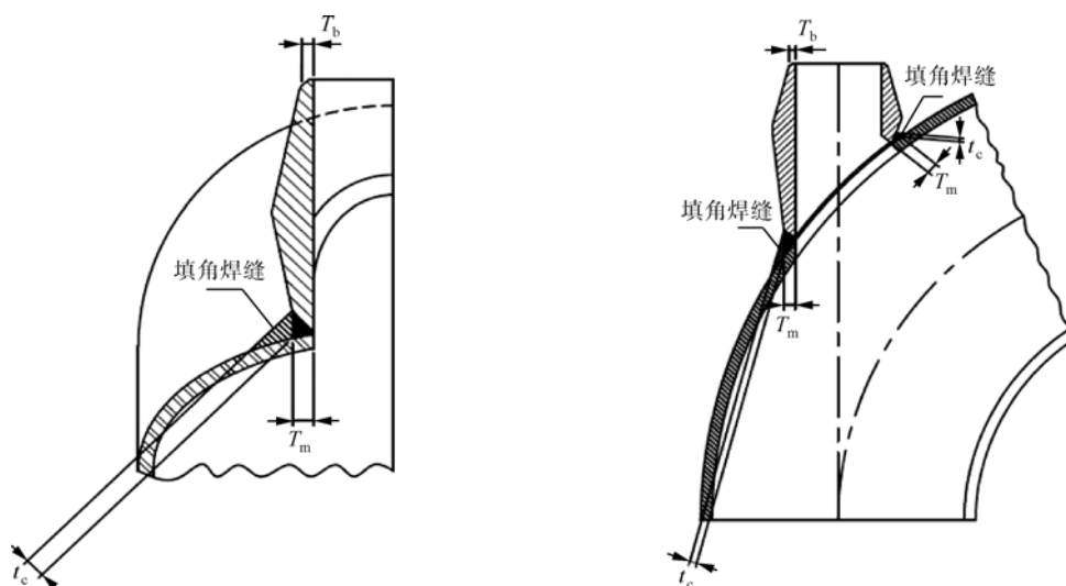
g) 弯头支管座纵横剖面
