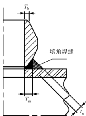
c) 带补强板的安放式焊接支管
