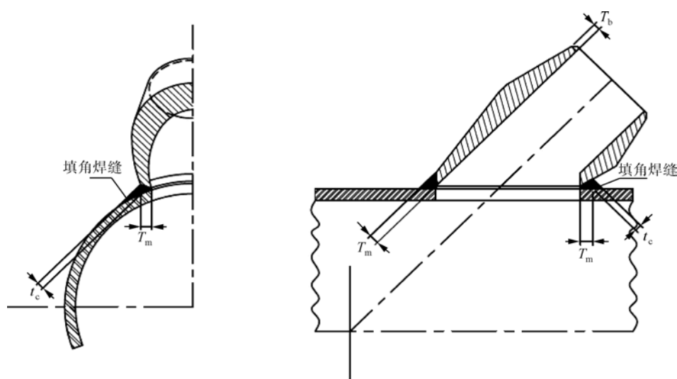
f) 斜接支管座纵横剖面
